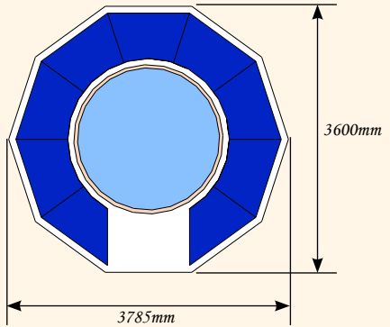
12ft x 12ft
